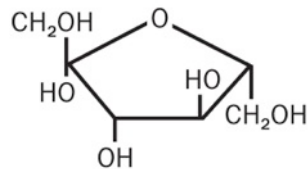
Fructose
